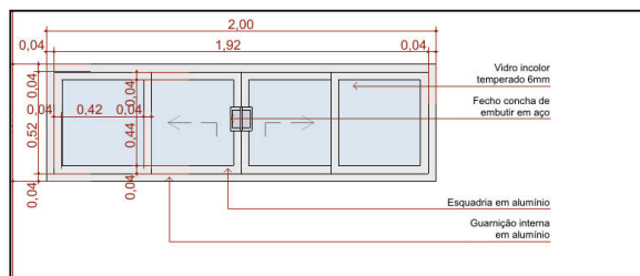
DETALHAMENTO DE JANELAS · PROJETO EXECUTIVO
